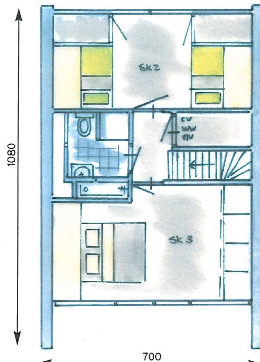
Plattegrond verdieping
